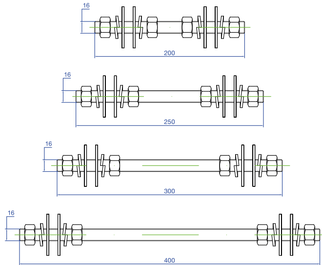
Plano perno tipo "esparrago"
